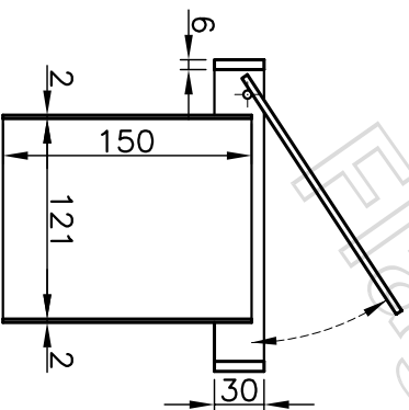
SECCIÓN CONJUNTO
