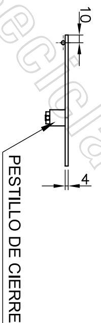
ALZADO TAPA
