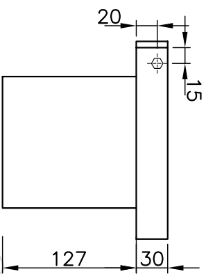
ALZADO EXTRAIBLE
